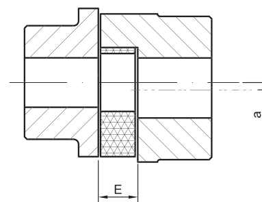
Désalignement radial
